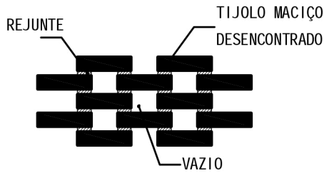
SUMIDOURO DETALHE DA ALVENARIA
